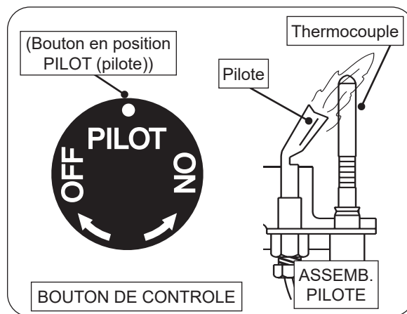
Fig. 53-1 Éclairage pilote
