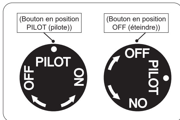
Fig. 54-2 Arrêt manuel
