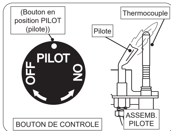
Fig. 43-1 Éclairage pilote
