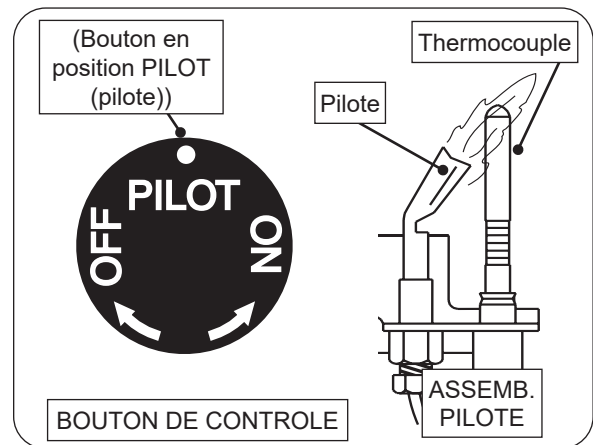
Fig. 43-1 Éclairage pilote
