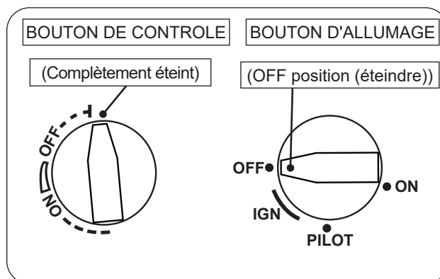
Fig. 51-2 Arrêt manuel
